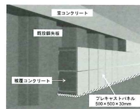
「ストパネ工法」の構造概念図
